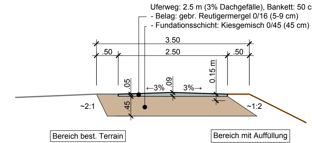
Normalprofil Uferweg 1:50
